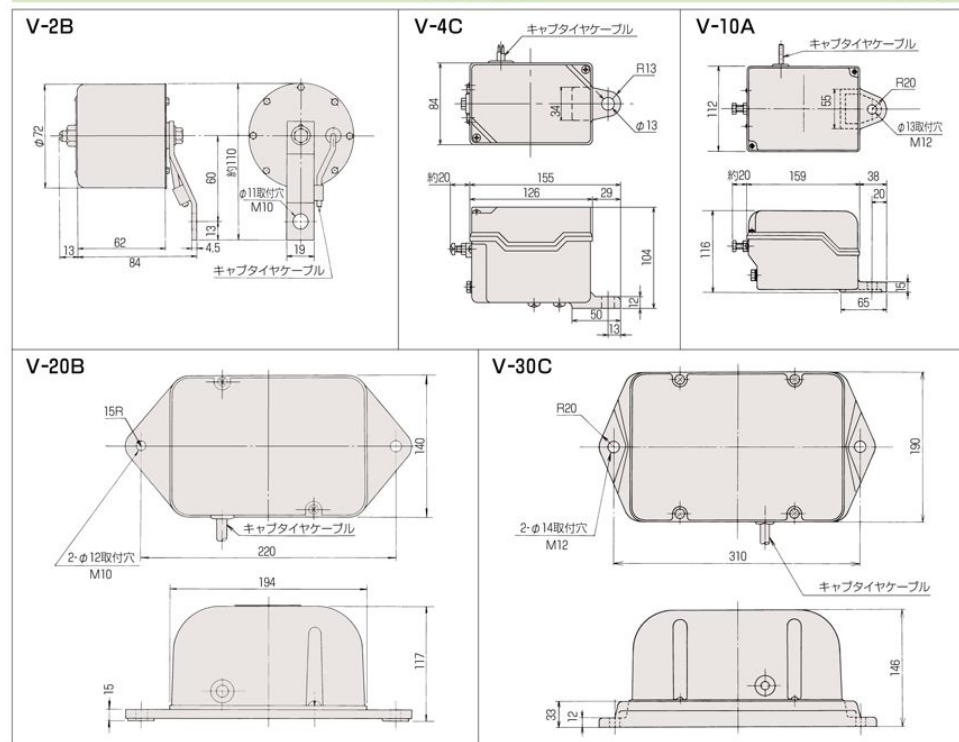
外形寸法図
