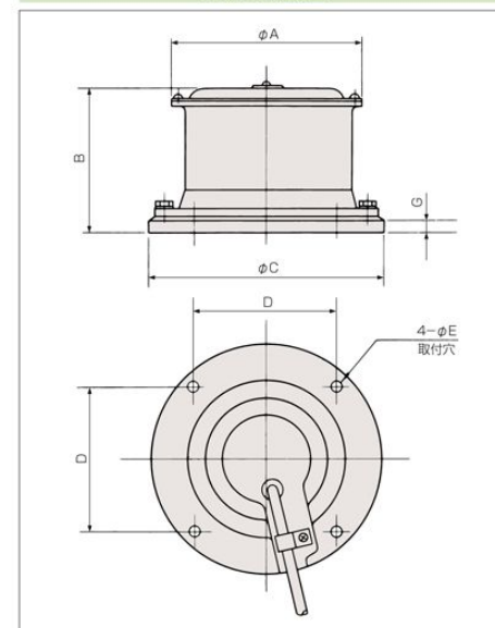
●寸法表
