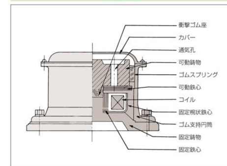
構造図
